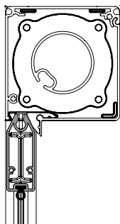
Caisson droit
